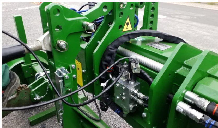
Figura 1.6.b - Esempio di collegamento delle elettrovalvole
