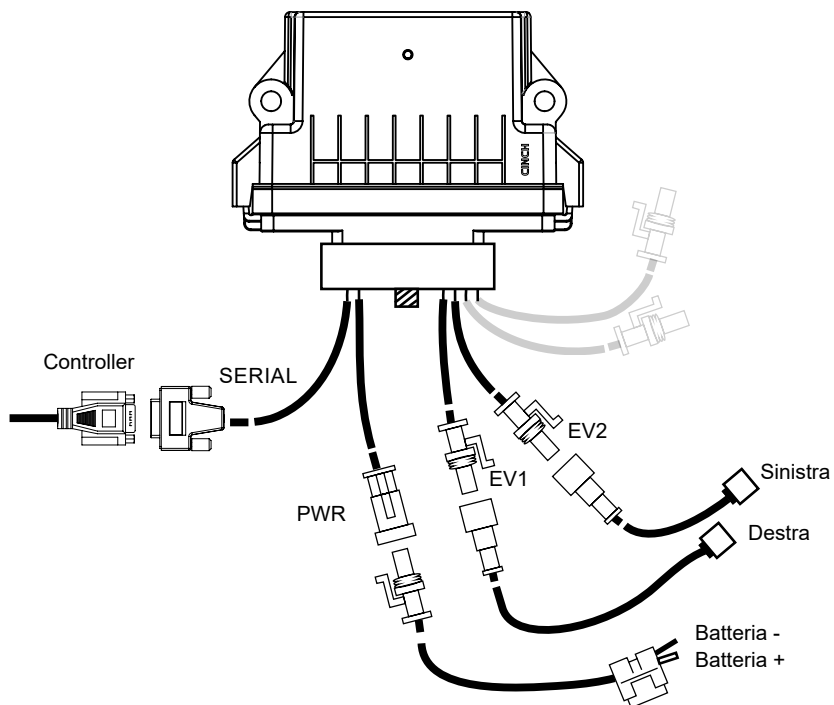
Figura 1.6.a - Schema collegamento ECU Dataseed
